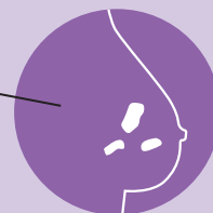
borstkanker
